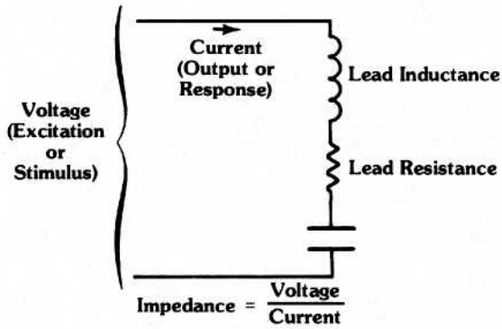
a) Actual impedance of a real capacitor
