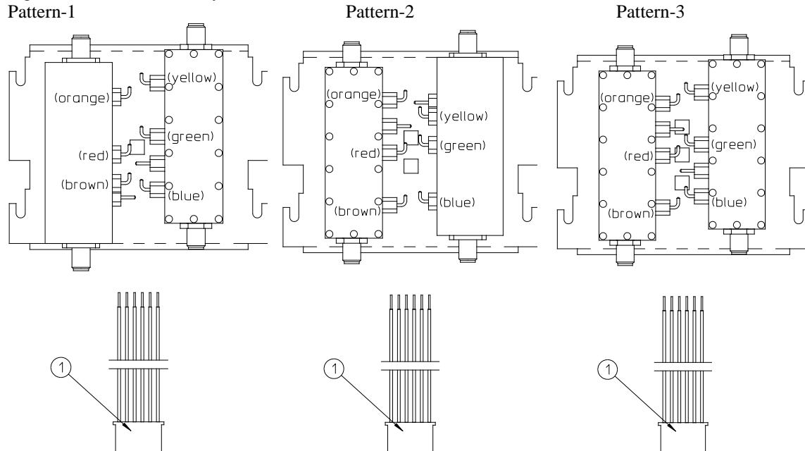
Figure 12-7. ATT Assembly Parts 2/2
